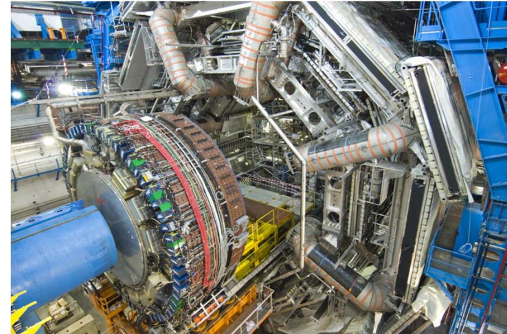
ATLAS Detector am LHC
