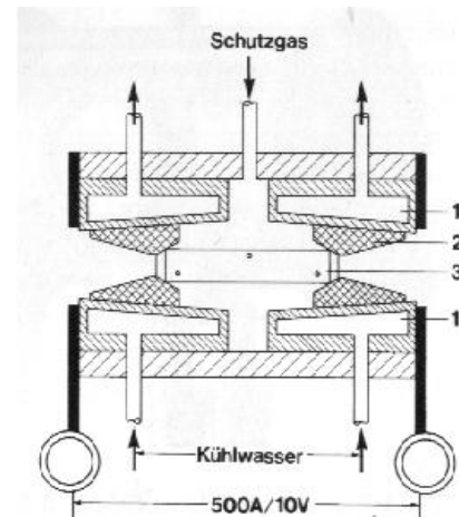
Abb. Graphitrohrofen von Perkin-Elmer
