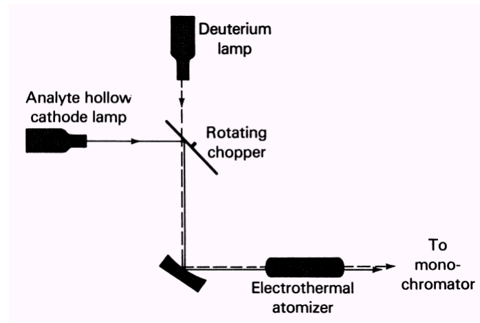
Abb. Schema eines Untergrundkorrektursystems für Kontinuumsstrahler.
