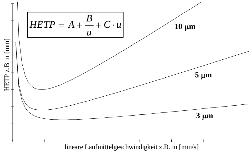
typische van-Deemter HETP/u-Kurven und Trägerpartikeldurchmesser
