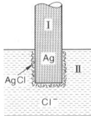
Ionenelektrode zweiter Art
