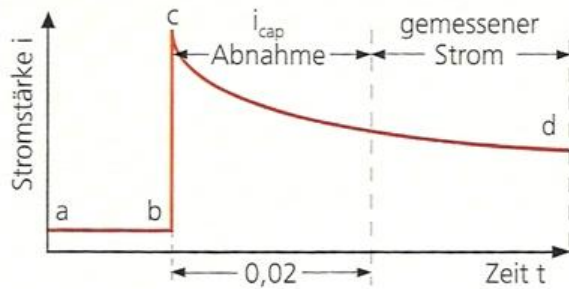
2. Strom-Zeit-Kurven
