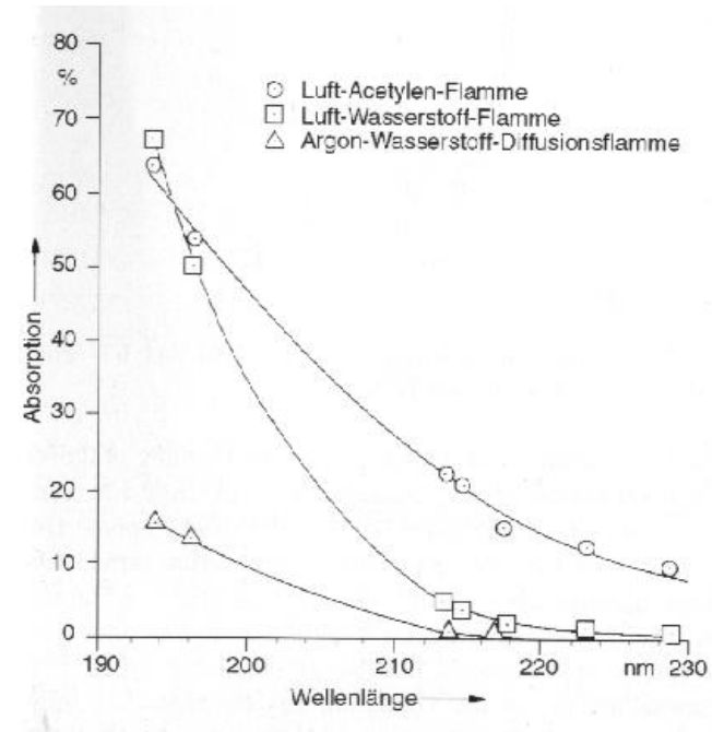
Abb. Eigenabsorption einiger Flammen (Argon-Wasserstoff-Diffusionsflamme: keine Zugabe von Sauerstoff (O 2 diffundiert von aussen in die Flamme ein))
