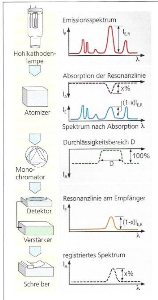
Abb. 6.3 Messprinzip der Atomabsorptions-Spektrometrie.
