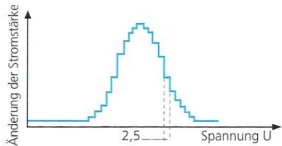
Abb. 4.20 Vergleich von pulse - und differenzieller pulse -Polarographie.
