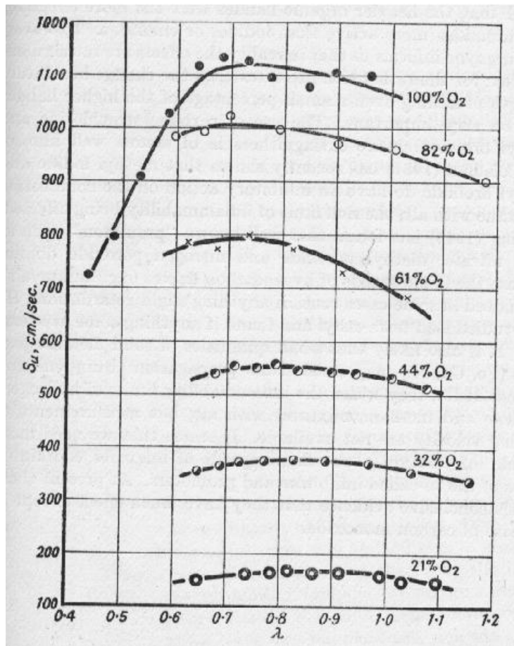
Abb. Änderung der Brenngeschwindigkeit als Funktion des Brenngas/Oxidants-Verhältnisses ( \lambda ) (1=stöchiometrisch) und des Sauerstoffgehaltes des Oxidants (aus Flames, Gaydon, Wolfhard, 1953)
