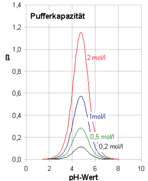
Abb.(unten) Pufferkapazität von Essigsäure/Acetatsystemen unterschiedlicher Konzentrationen
