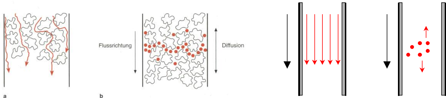
Abb. Schematische Darstellung der Eddy-Diffusion (a) und der Longitudinaldiffusion (b) bei gepackten Säulen (links) und Kapillarsäulen (rechts)
