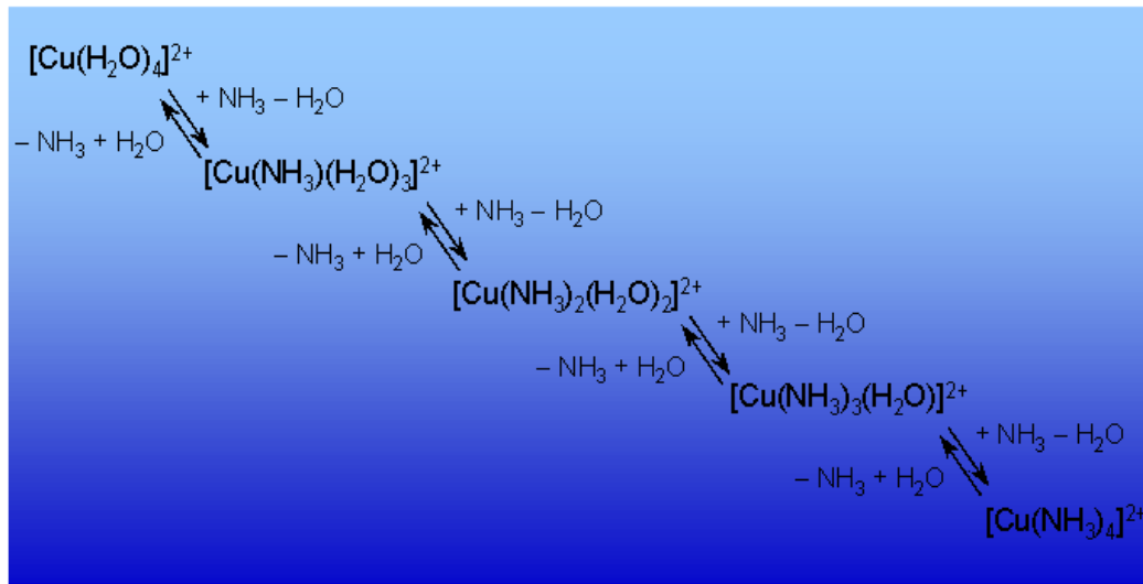
Abb. Ligandenaustauschreaktionen
