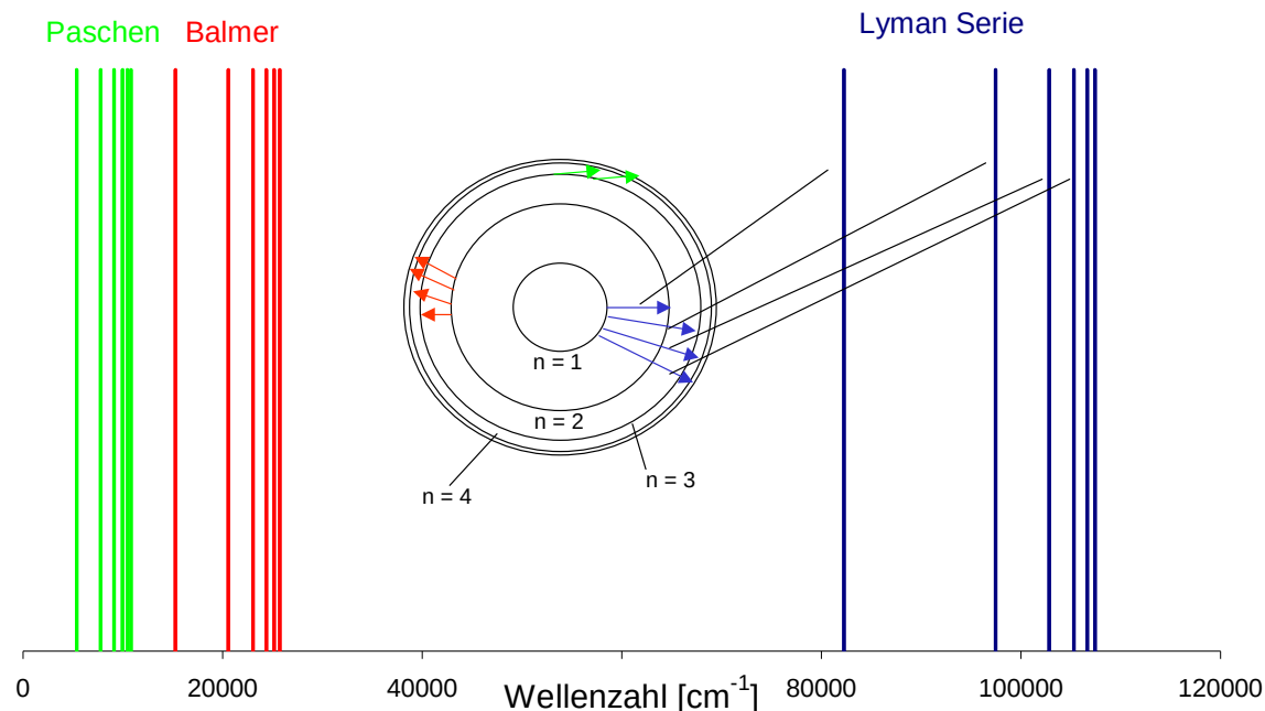
Abb. Linienspektrum des Wasserstoffs als Funktion der Wellenzahl ( \nu' ) (welche proportional zur Energie ( E = h \cdot c \cdot \nu' ) der absorbierten Strahlung ist)
