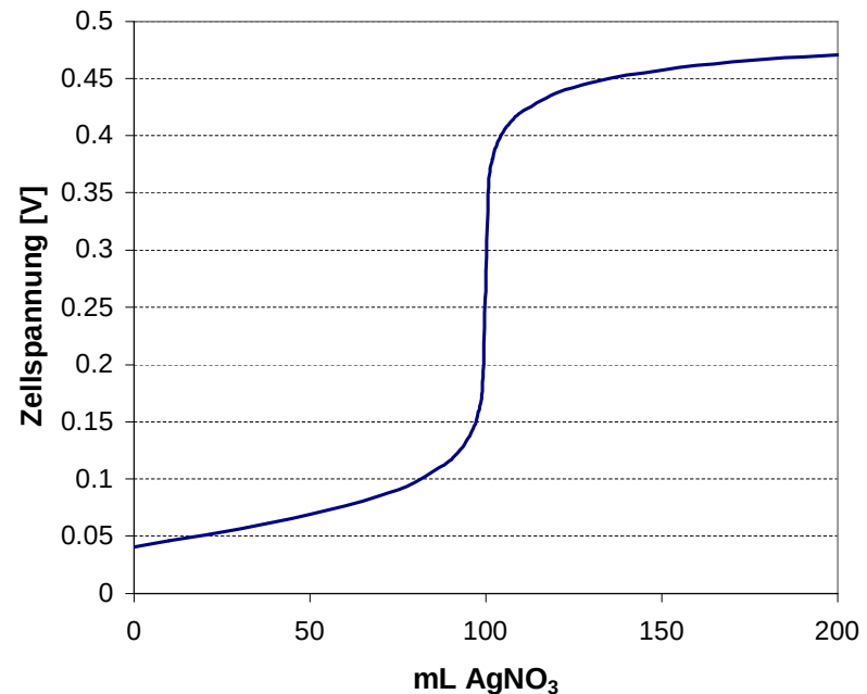
Abb. Titrationskurve der oben diskutierten Titration
