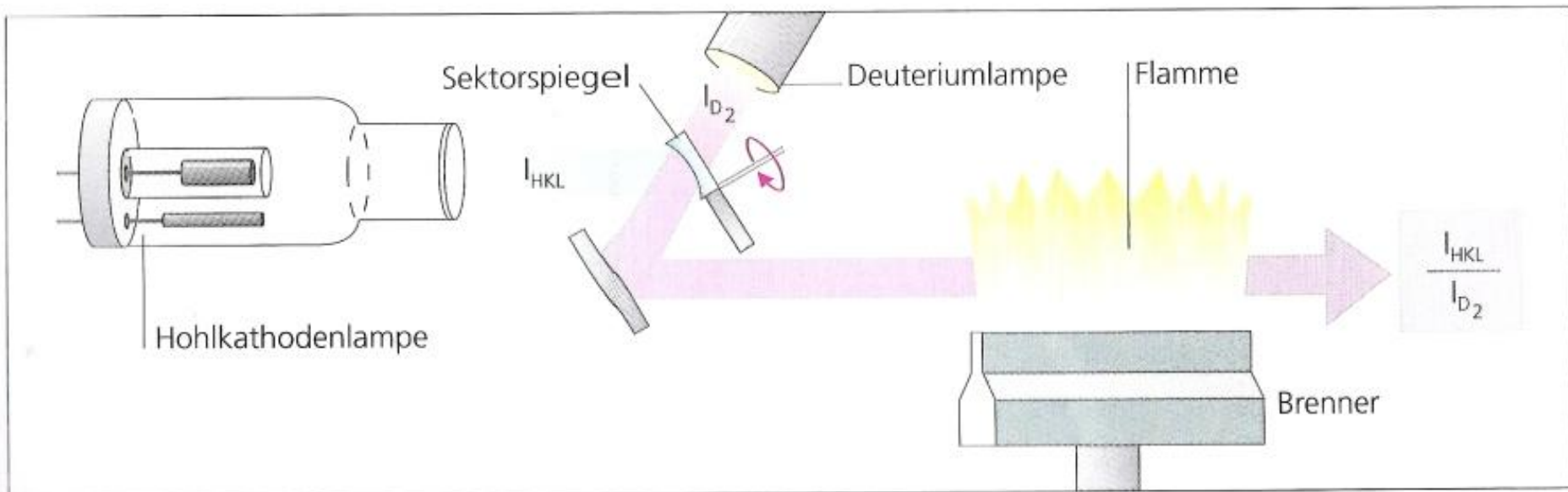
Abb. 6.9 Funktionsweise eines Deuterium-Untergrundkompensators
