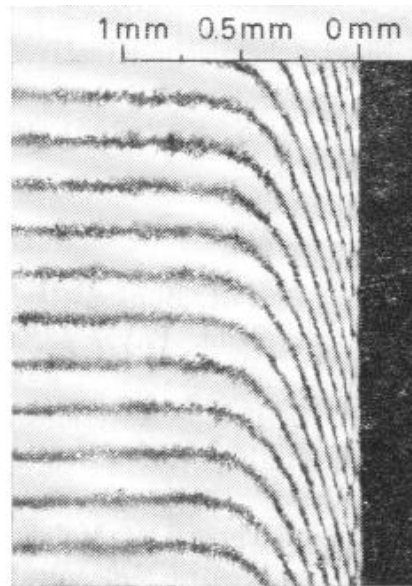
Abb. Sichtbarmachung der kathodischen Diffusionsschicht bei der Elektrolyse von \text{CuSO}_4 (links – stromlos, rechts – bei Stromfluß)
