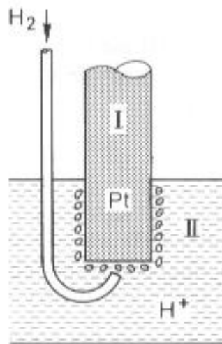
Redoxelektrode (heterogenes System; Gaselektrode)
