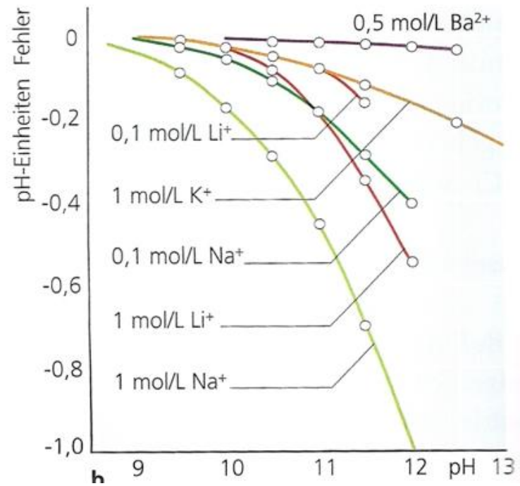
Abb. Alkali-Fehler von pH-Glaselektroden
