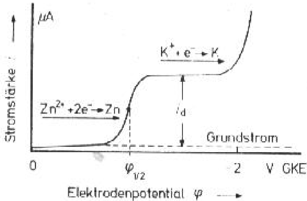
Abb. Polarogramm einer Zink-Ionen (Depolarisator) enthaltenden Lösung (KCl als Leitelektrolyt), i_d = Diffusionsgrenzstrom der Zinkionen, E_{1/2} Halbstufenpotential (gegen GKE (=SCE) gesättigte Kalomel-Elektrode)
