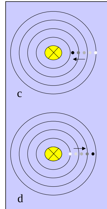
Abb. Ursache der Dopplerverbreiterung in der AAS.
