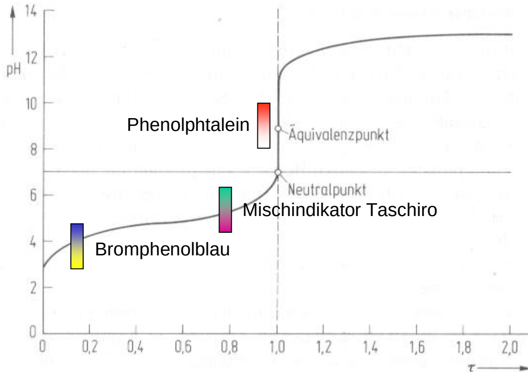
Abb. Titration von 0.1 M Essigsäure mit 10 M Natronlauge - Indikatoreauswahl
