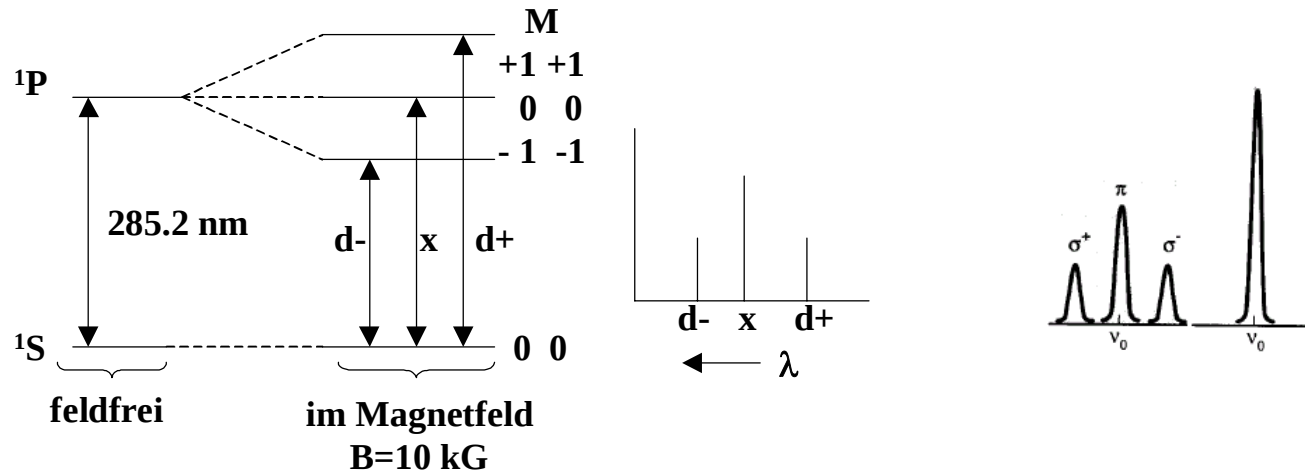
Abb. Zeeman-Effekt – Energieniveaus in starken Magnetfeldern
