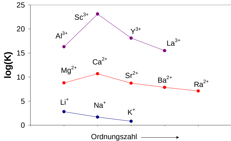
Abb. Stabilitätskonstanten für Metall-EDTA-Komplexe
