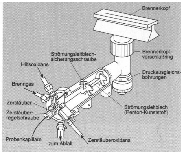
Abb. Laminarstrombrenner
