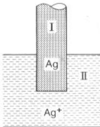
Ionenelektrode erster Art
