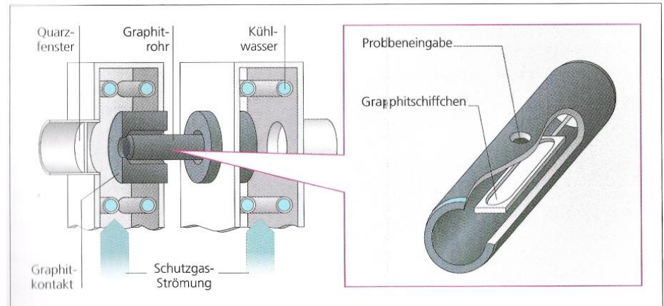
Abb. 6.6 Aufbau eines Graphitrohrofens – Graphitrohr mit IL'vov-Plattform.
