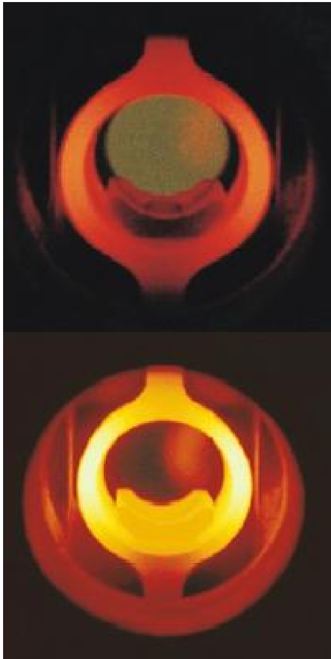
Abb. 6.6 Aufbau eines Graphitrohrofens – Graphitrohr mit IL'vov-Plattform.
