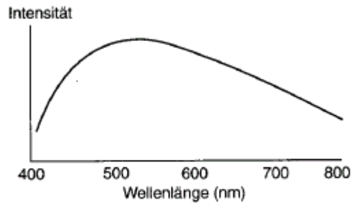
Emissionsspektrum einer Halogenlampe
