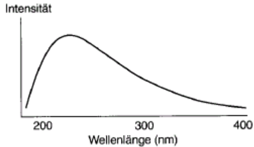
Emissionsspektrum einer Deuteriumlampe
