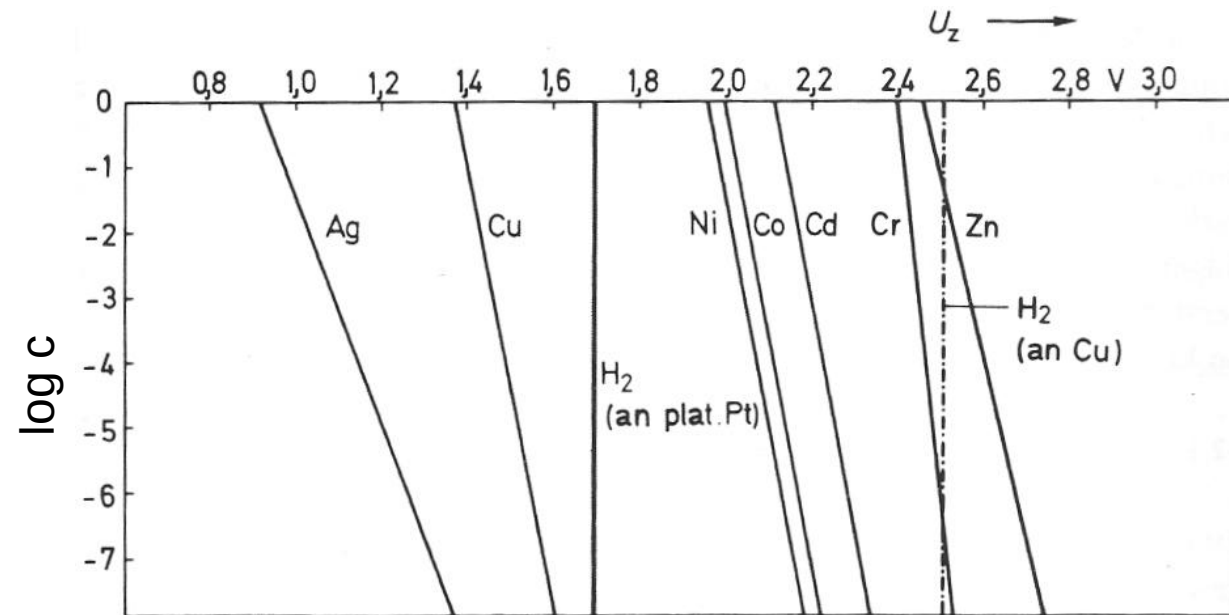
Abb. Zersetzungsspannung von Metallsulfaten in 0,5 molarer Schwefelsäure
