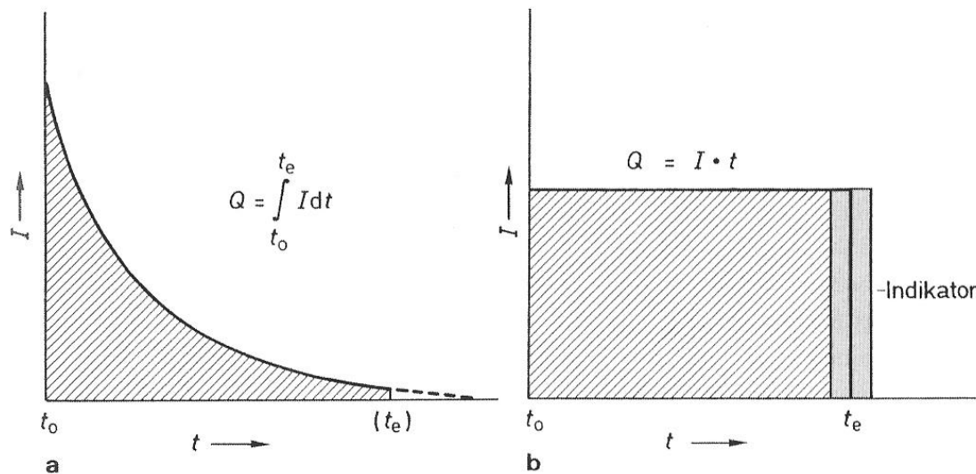
Abbildung 54 a Potenziostatische Coulometrie, b galvanostatische Coulometrie.
