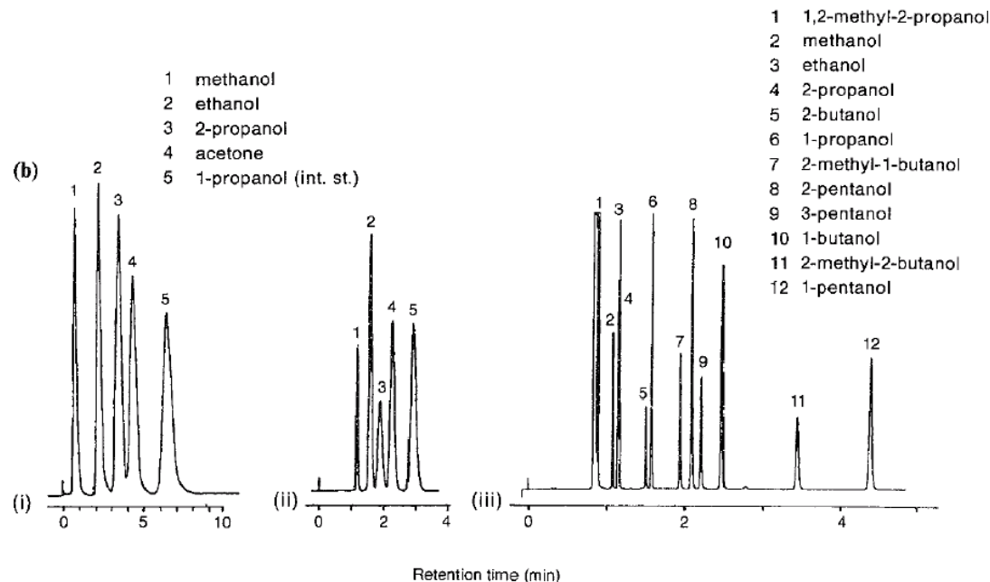
Abb. Vergleich der Trennung auf einer gepackten Säule (links) (2 m Länge, 3 mm i.D.), einer wide bore Kapillarfilmsäule (Mitte) (10 m Länge, 0.53 mm i.D. FD 2 µm) und einer "Standard"-Kapillardünnsäule (rechts) (25 m Länge, 0.25 mm i.D., FD 0.25 µm)
